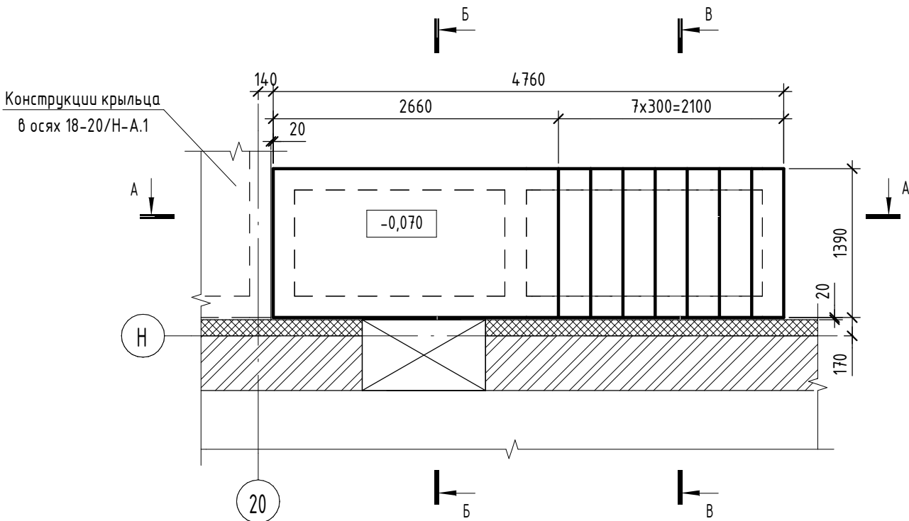
Схема расположения входной группы в/о 20/Н на отм. -0,070
