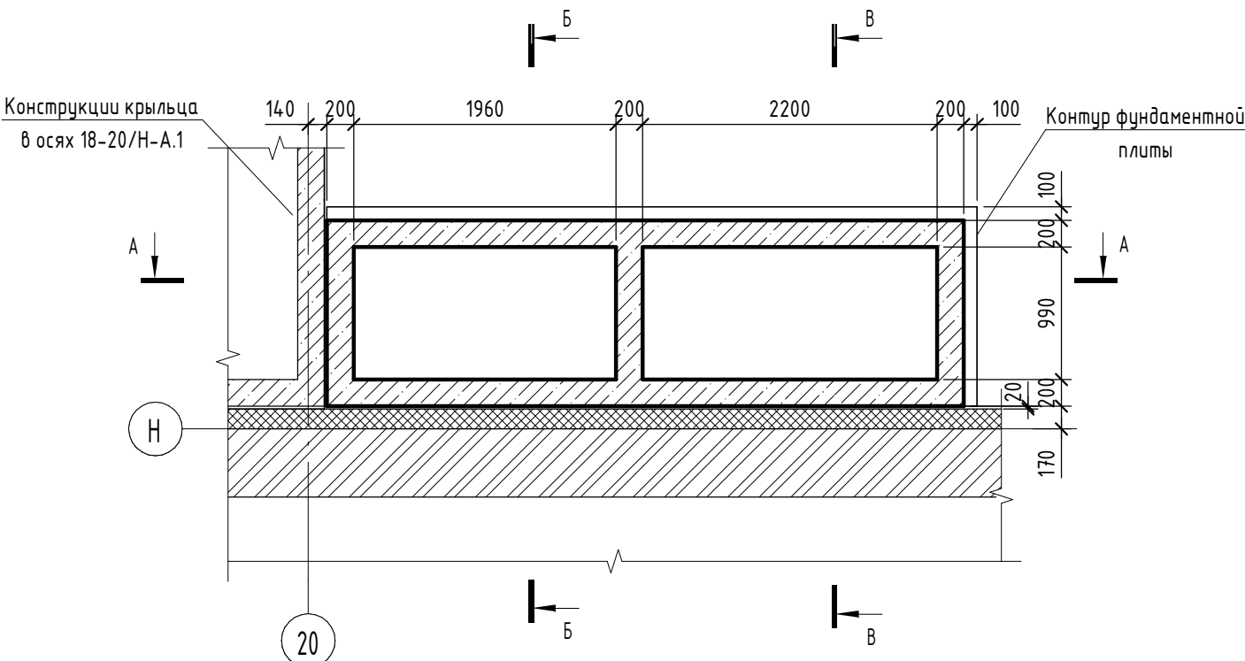
Схема расположения стен входной группы в/о 20/Н на отм. -1,700
