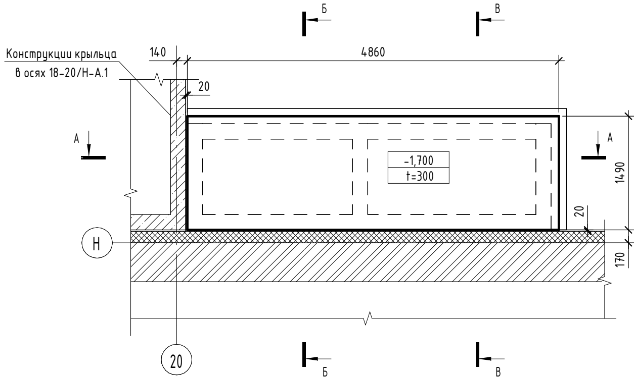
Схема расположения фундаментной плиты входной группы в/о 20/Н на отм. -1,700
